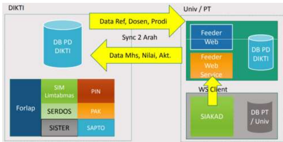
Gambar 5.1 Arsitektur PD-Dikti
